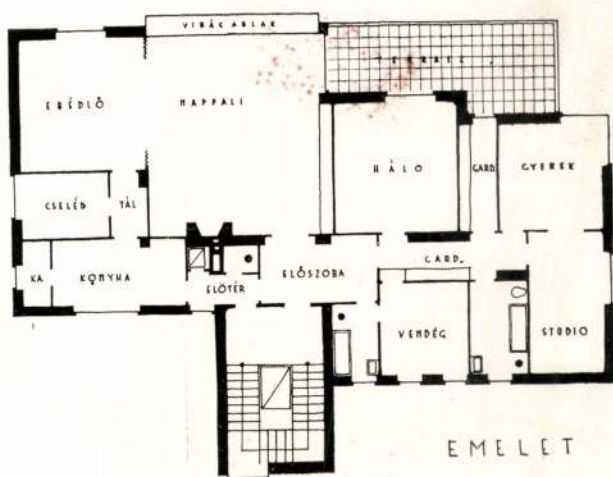
POGÁNY MÓRIC: HÁROMLAKÁSOS CSALÁDI HÁZ AZ ÁFONYA-UTCÁBAN M. POGÁNY: EINZELHEITEN EINES FAMILIENWOHNHAUSES — DÉTAILS D'UNE MAISON DE FAMILLE — DETAILS OF A DWELLING-HOUSE
